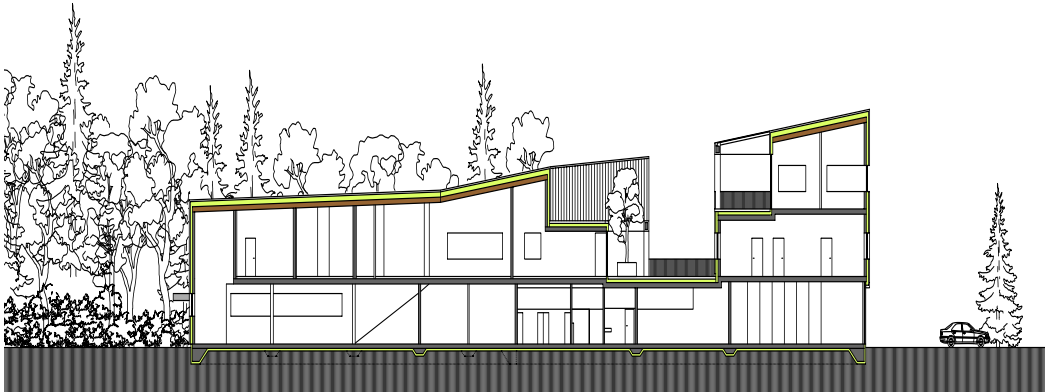
Schnitt
